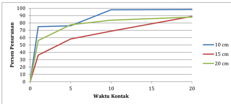
Gambar 4. Presentase Penurunan Jumlah Bakteri pada Air Minum akibat Penyinaran Ultra Violet menurut Ketebalan dan Waktu Kontak
